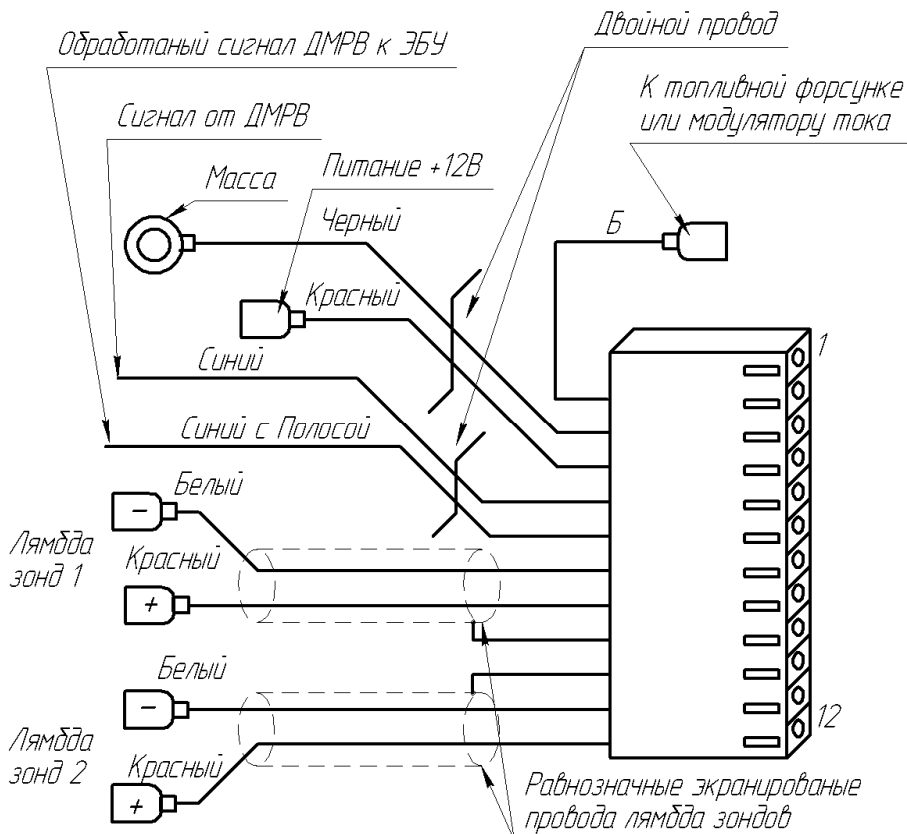
Рисунок 3.2. Назначение проводов.
