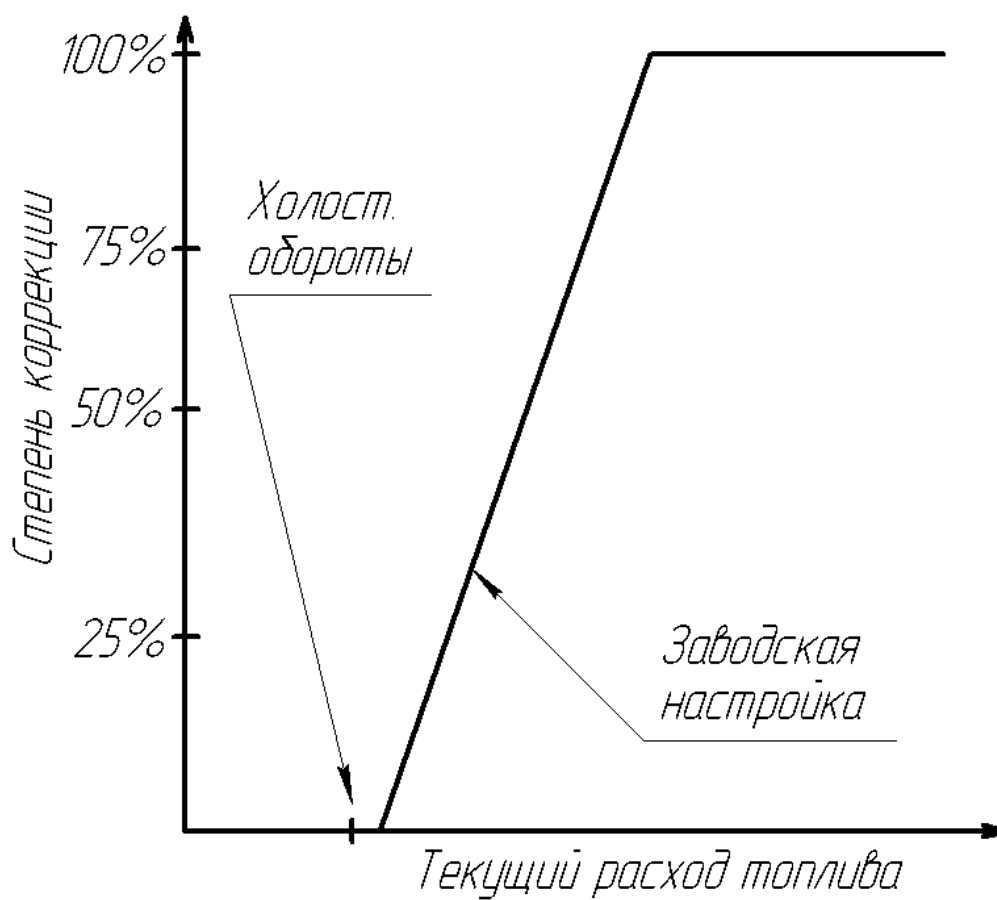
Рисунок 3.6. Зависимость степени коррекции от текущего расхода топлива.
