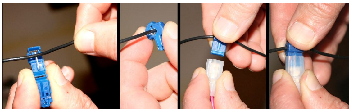
Рисунок 3.4. Методика подключения проводов при помощи быстрых соединителей.
