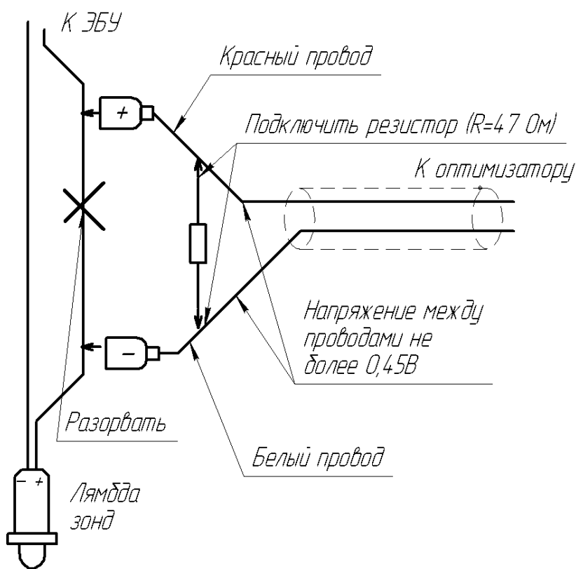
Рисунок 3.3. Схема подключения оптимизатора к циркониевому лямбда зонду при втором способе подключения.
